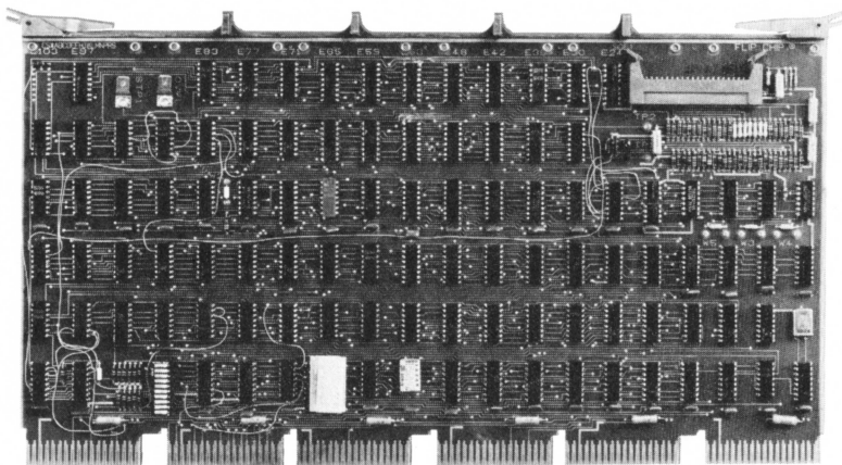
KW11-K
